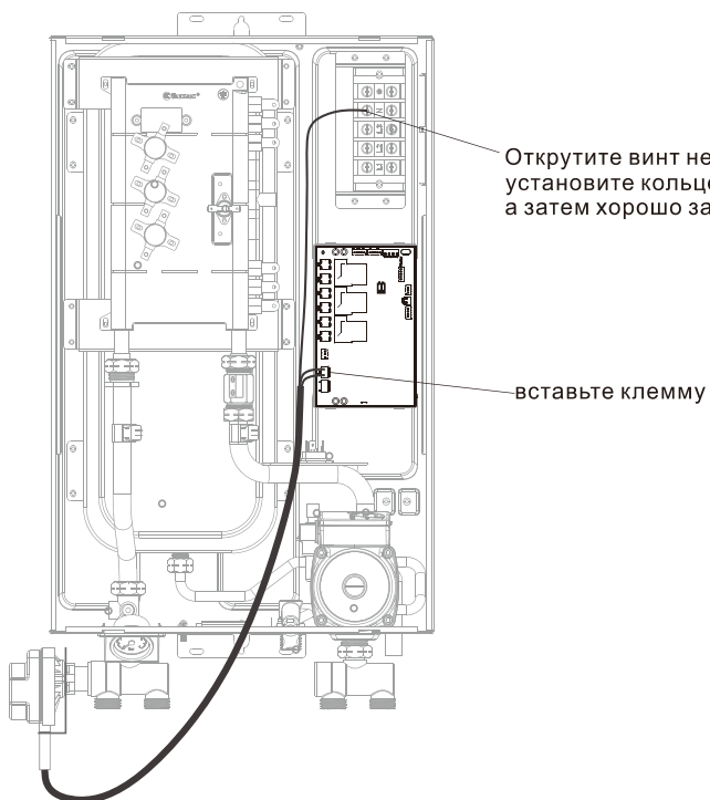
Рис. 16. Подключение трехходового клапана
